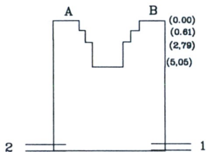
Šulinio pjūviai
