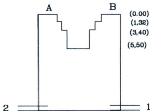
Šulinio pjūviai
