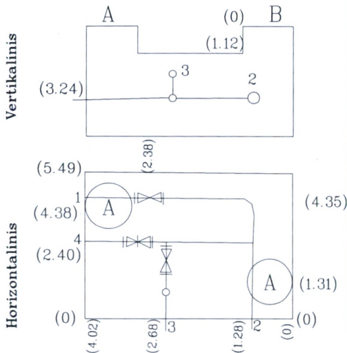
Šulinio pjūviai :
