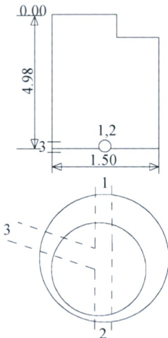
Šulinio pjūviai
