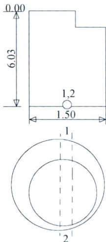
Šulinio pjūviai
