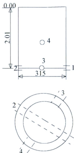
Šulinio pjūviai
