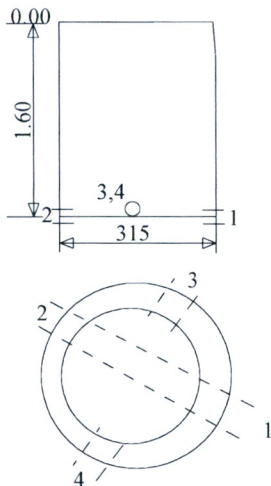
Šulinio pjūviai
