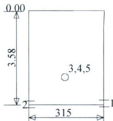
Šulinio pjūviai
