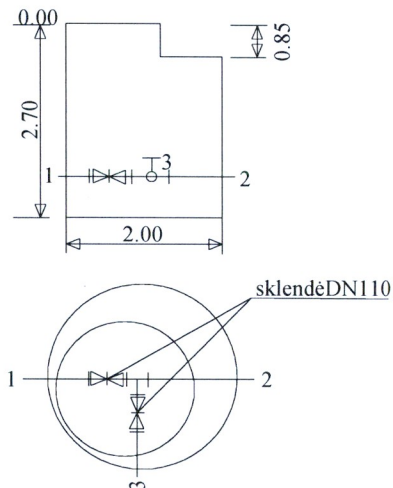
Šulinio pjūviai
