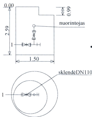
Šulinio pjūviai
