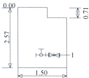
Šulinio pjūviai
