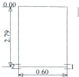
Šulinio pjūviai
