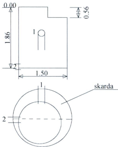
Šulinio pjūviai
