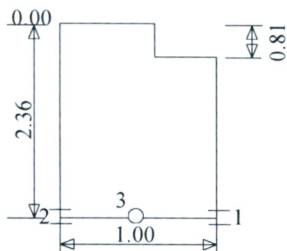
Šulinio pjūviai
