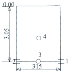
Šulinio pjūviai
