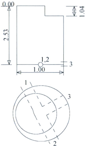
Šulinio pjūviai
