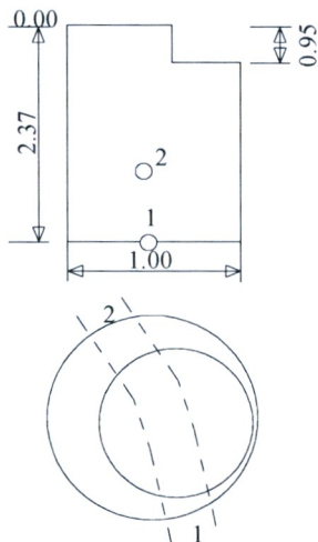
Šulinio pjūviai
