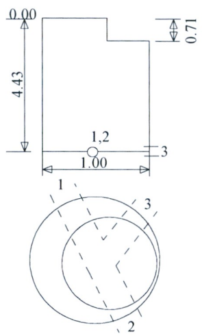
Šulinio pjūviai
