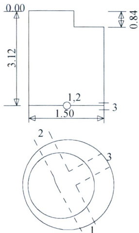
Šulinio pjūviai
