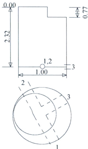
Šulinio pjūviai
