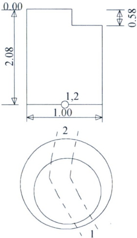
Šulinio pjūviai
