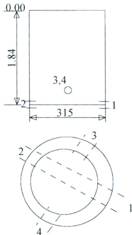
Šulinio pjūviai
