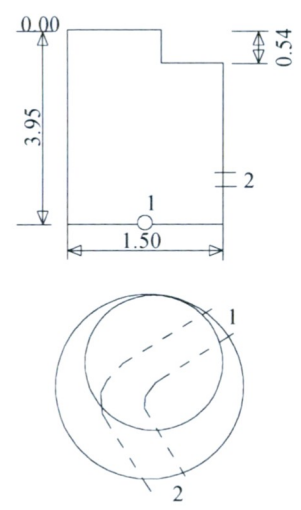
Šulinio pjūviai
