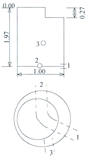
Šulinio pjūviai
