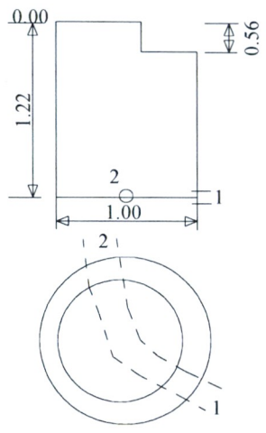
Šulinio pjūviai
