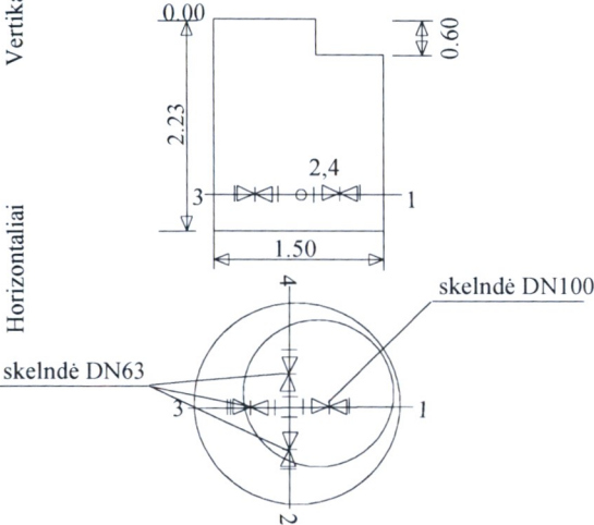
Šulinio pjūviai
