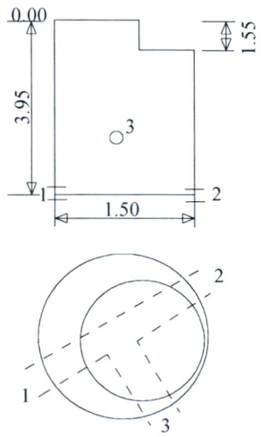
Šulinio pjūviai
