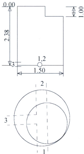
Šulinio pjūviai
