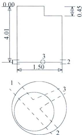
Šulinio pjūviai
