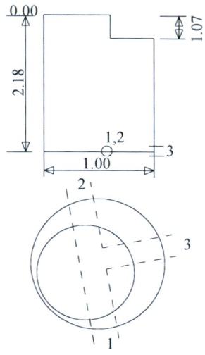
Šulinio pjūviai
