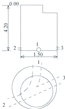
Šulinio pjūviai
