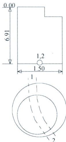
Šulinio pjūviai
