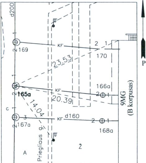
Pririšimo brėžinys
