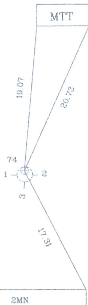
Pririšimo brėžinys
