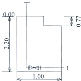
Šulinio pjūviai
