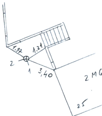
PRIRŪSIMO SCHEMA
